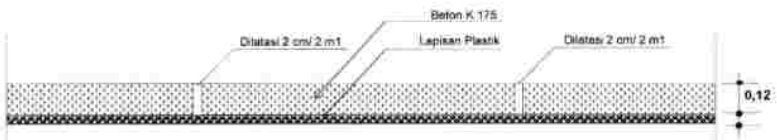
POTONGAN A - A
