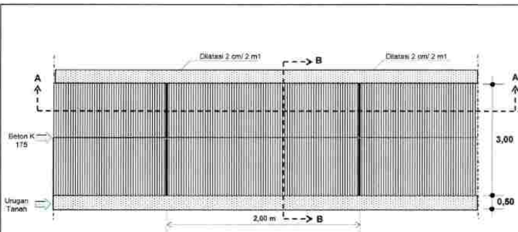
TAMPAK ATAS
