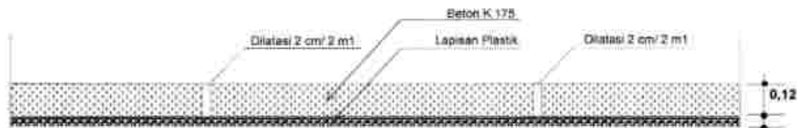
POTONGAN A - A
