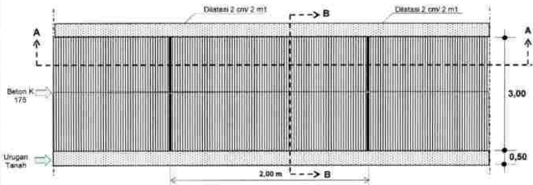
TAMPAK ATAS
