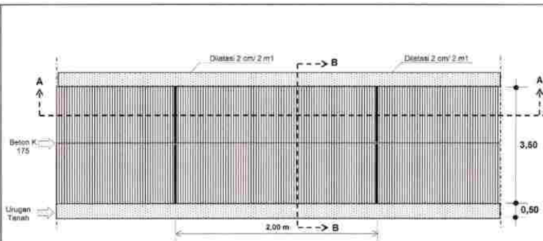
TAMPAK ATAS
