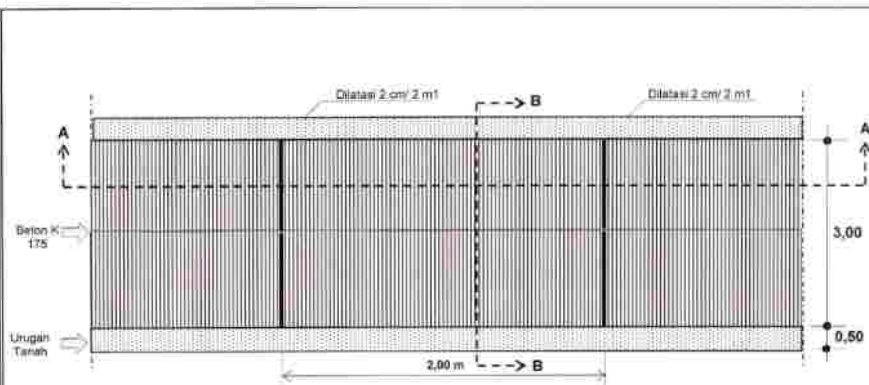
TAMPAK ATAS
